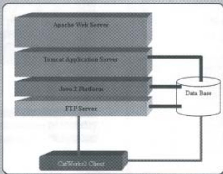
Catworks 的軟體架構圖
